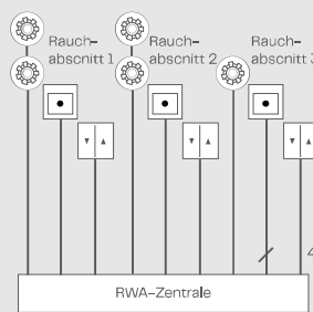
Typische Verkabelungsführung
